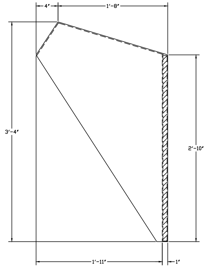
RIGHT ELEVATION
