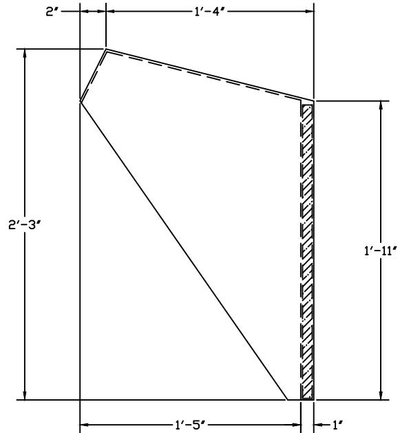
RIGHT ELEVATION
