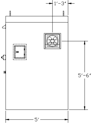
RIGHT ELEVATION
