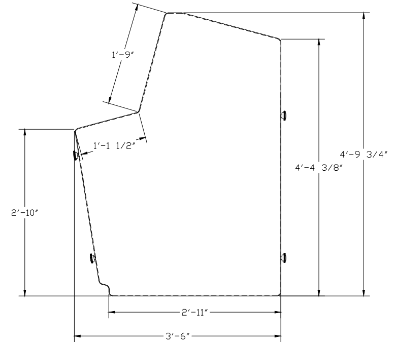
RIGHT ELEVATION
