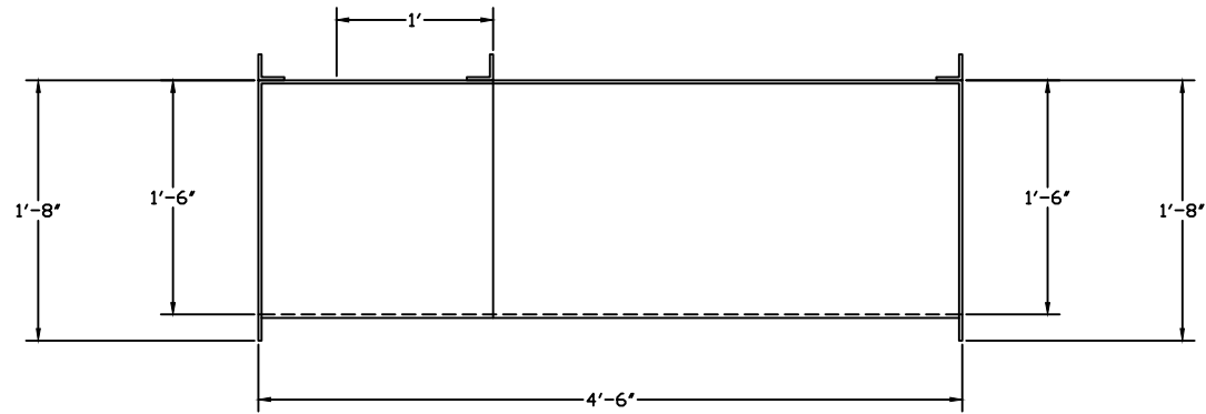
RIGHT ELEVATION
