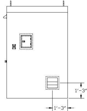
RIGHT ELEVATION
