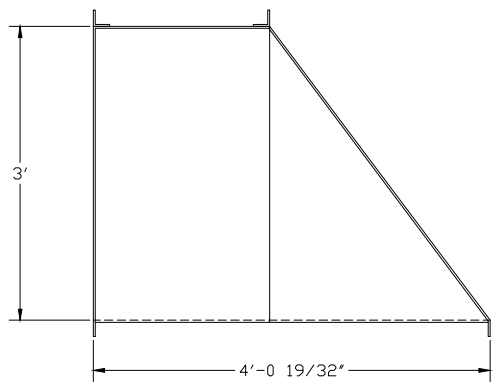
RIGHT ELEVATION
