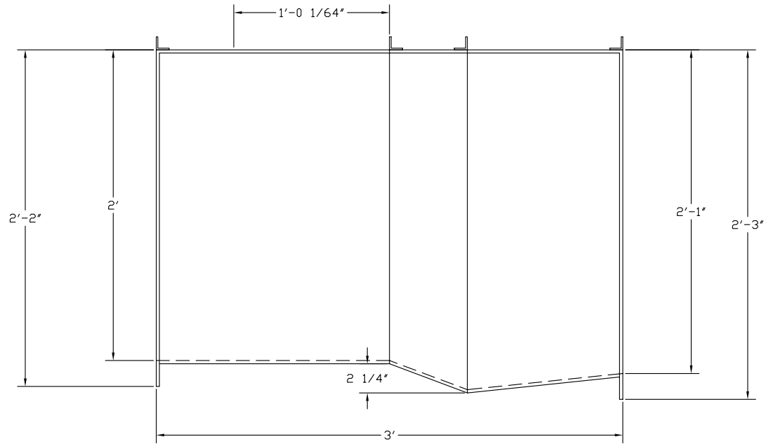
RIGHT ELEVATION
