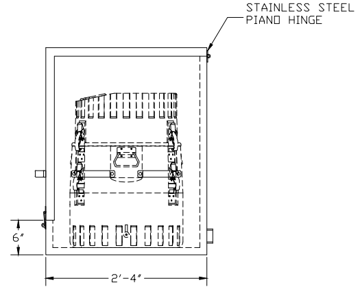
RIGHT ELEVATION
