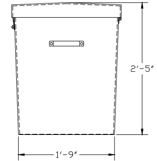
RIGHT ELEVATION
