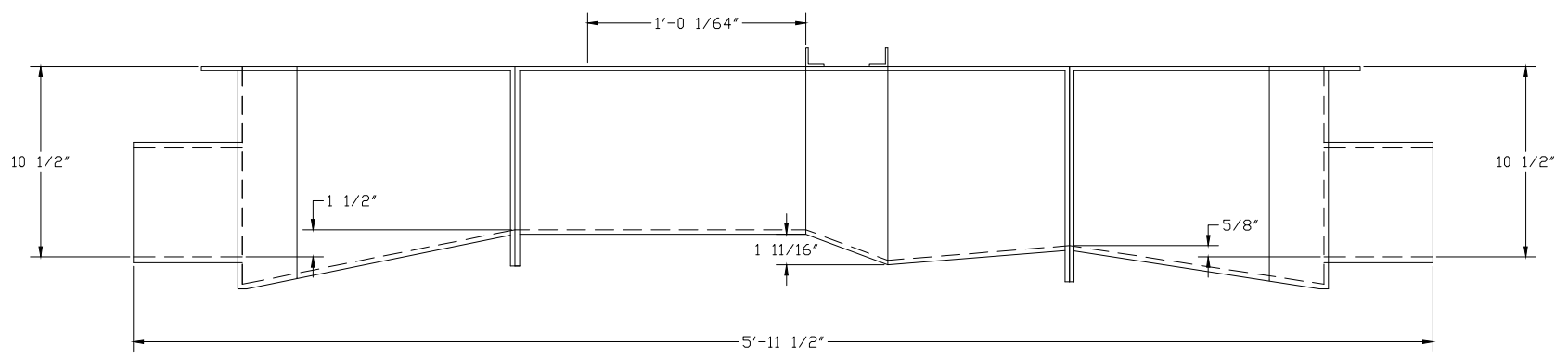
RIGHT ELEVATION
