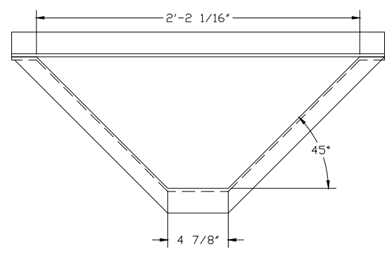
END ELEVATION
