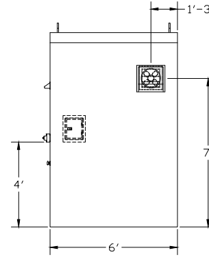
RIGHT ELEVATION
